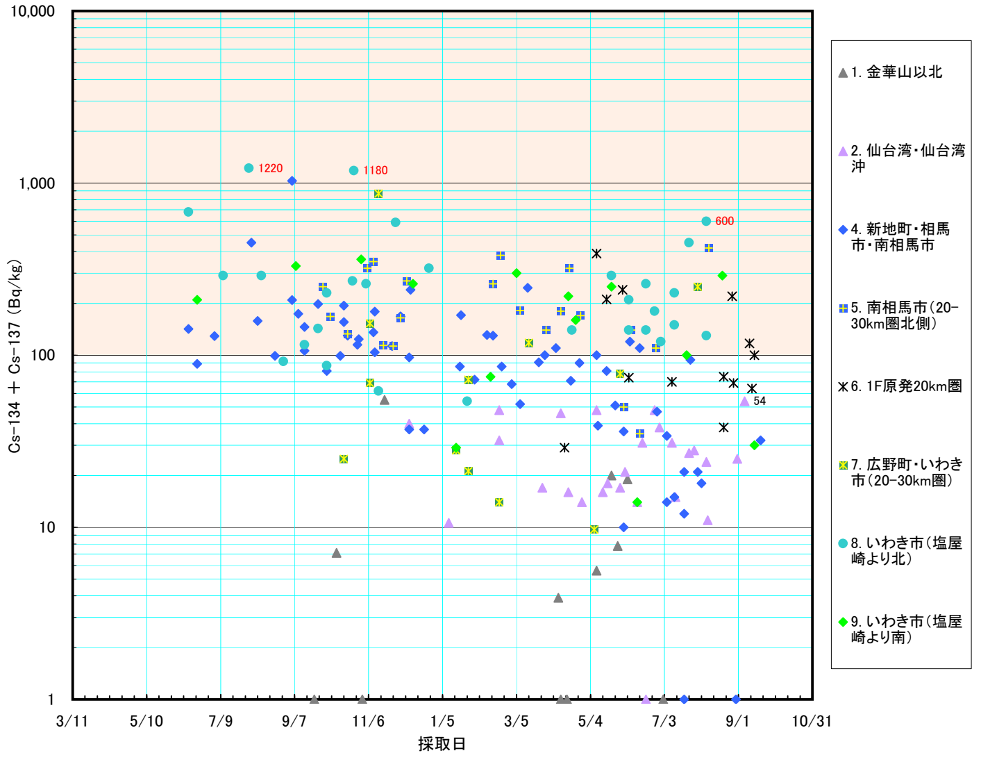
イシガレイ中のセシウム放射能濃度（福島以北、9/30公表分まで）
