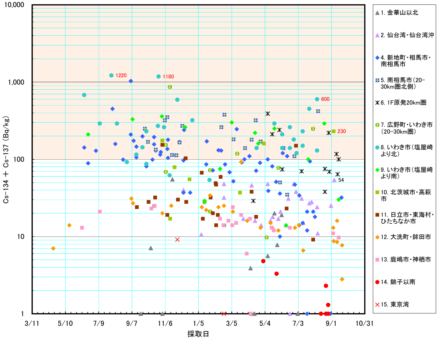
イシガレイ中のセシウムの放射能濃度 (9/30公表分まで)
