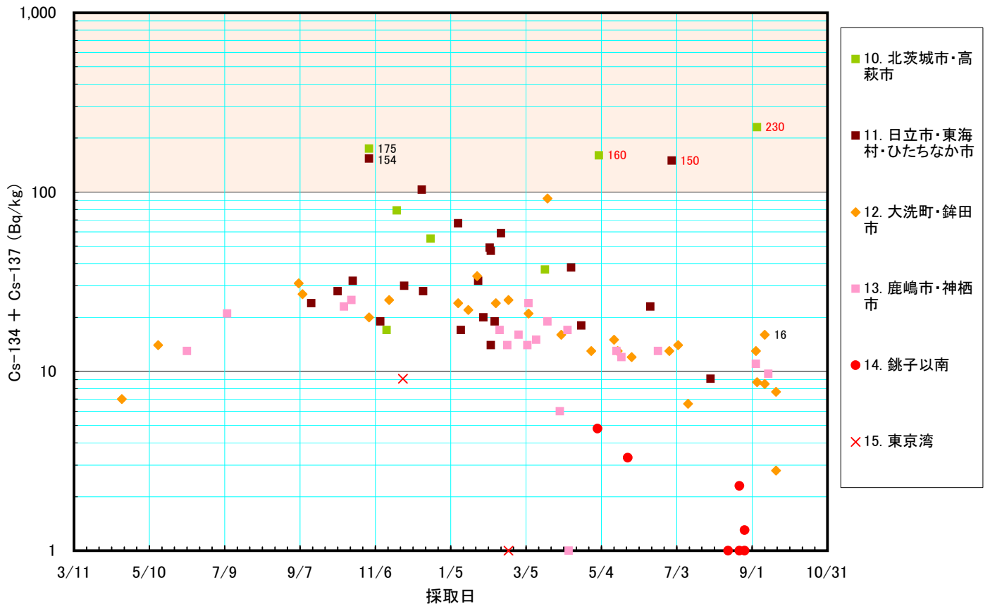
イシガレイ中のセシウム放射能濃度（茨城以南、9/30公表分まで）
