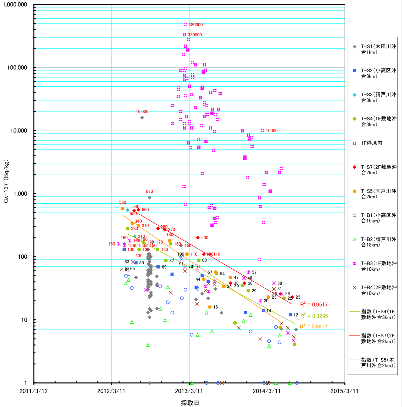
アイナメ中のCs-137の放射能濃度（東電 20km圏調査、2014/8/15公表分まで）
