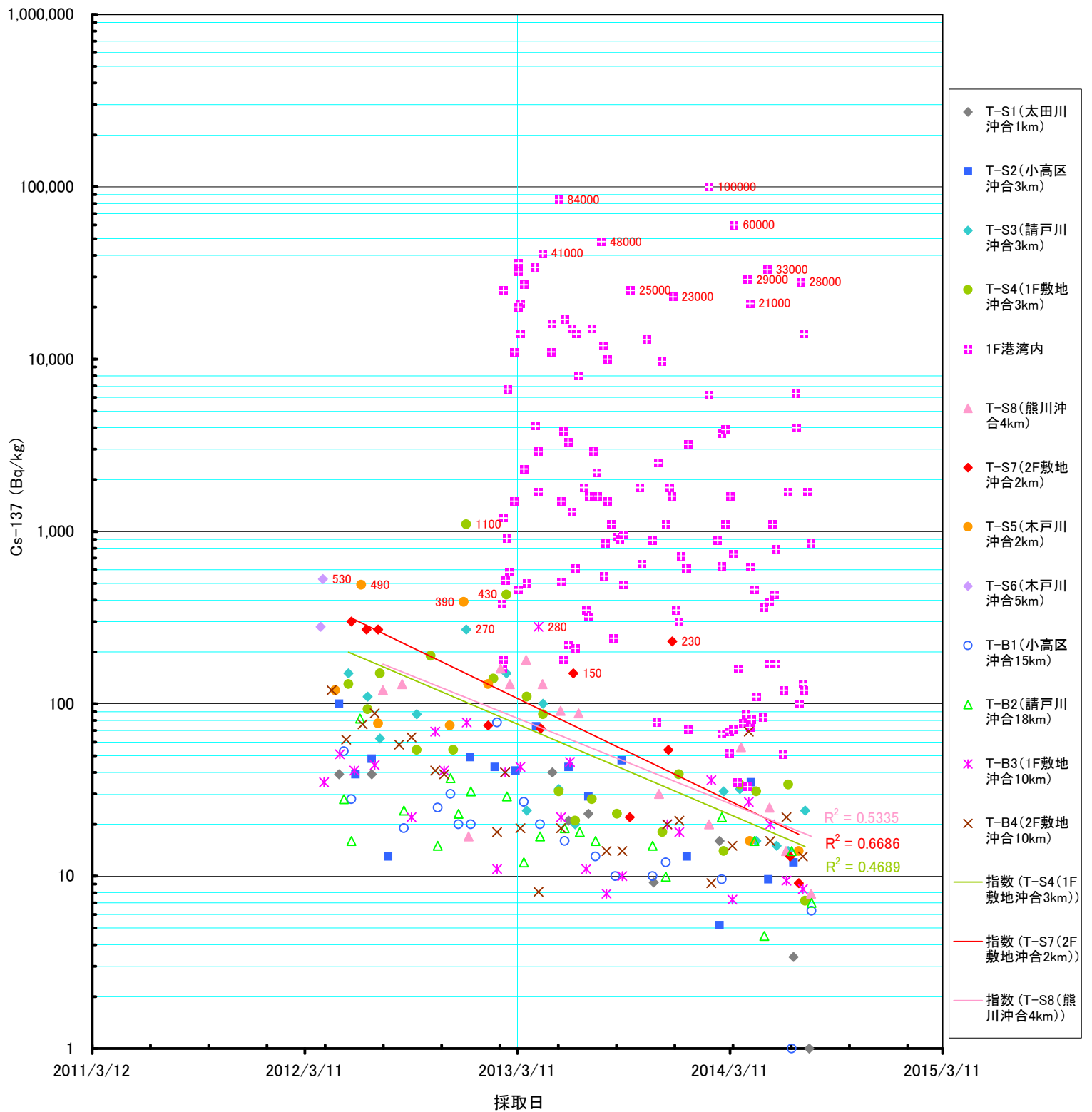
マコガレイ中のCs-137の放射能濃度（東電 20km圏調査、2014/8/15公表分まで）
