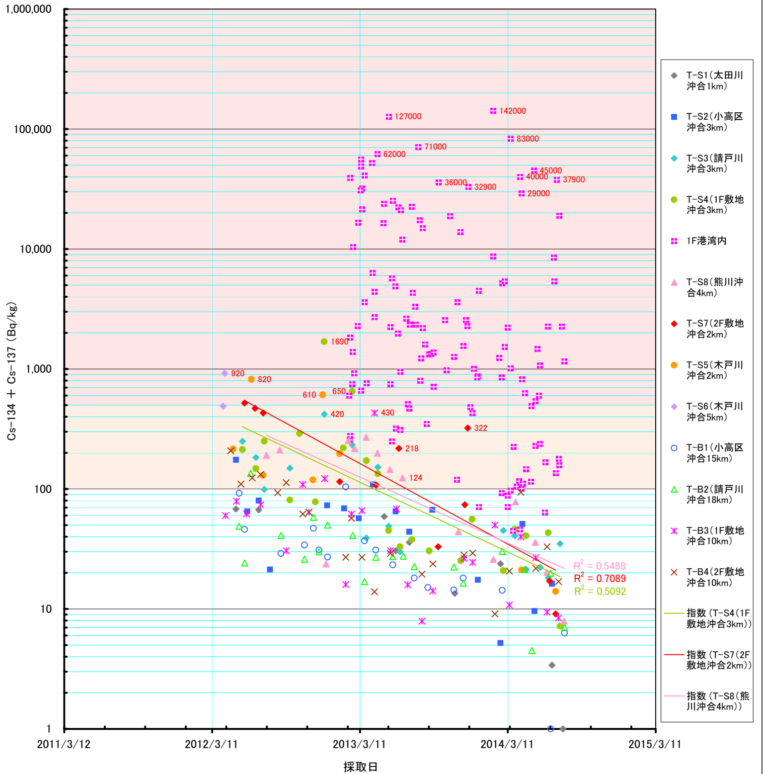
マコガレイ中のセシウム放射能濃度 (東電 20km圏調査、2014/8/15公表分まで)
