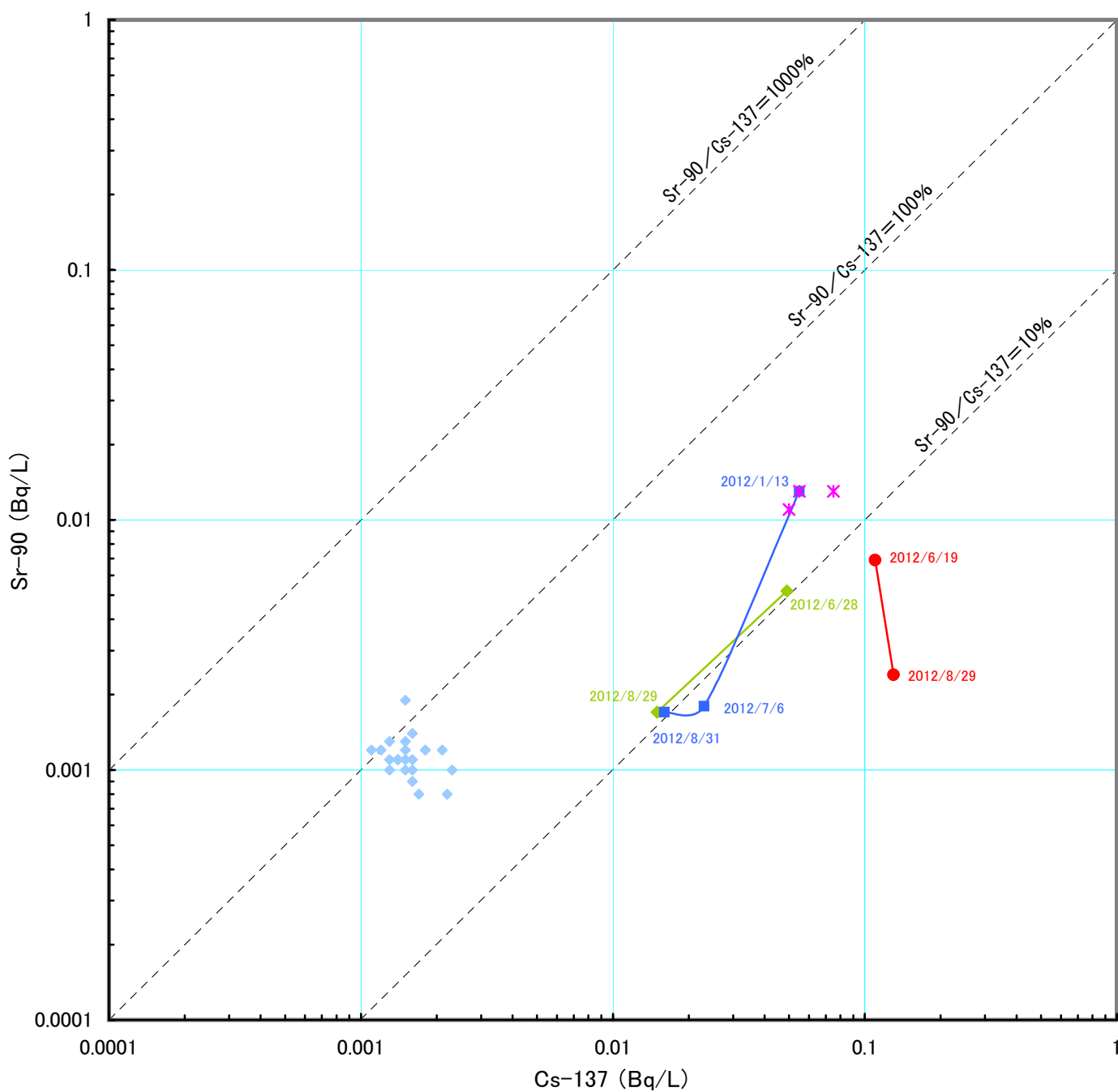
環境省調査による海水中のCs-137濃度とSr-90濃度の関係(定点における推移)
