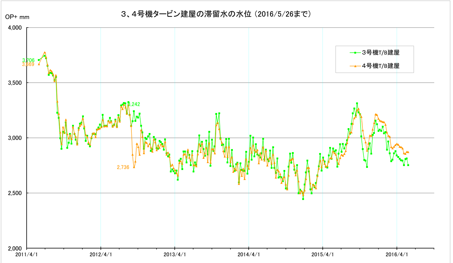
3号機、4号機タービン建屋の水位はほとんど連動しているが、2012年の9～10月にかけては大きくずれている。
