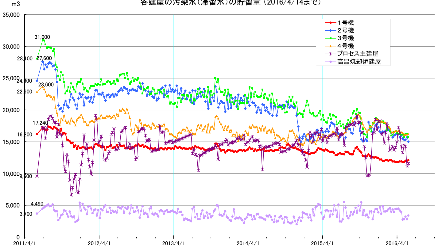
各建屋の汚染水(滞留水)の貯留量 (2016/4/14まで)
